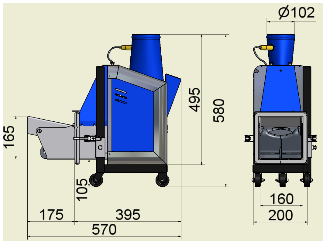
Figur 1. Mättskiss NH-brännare
